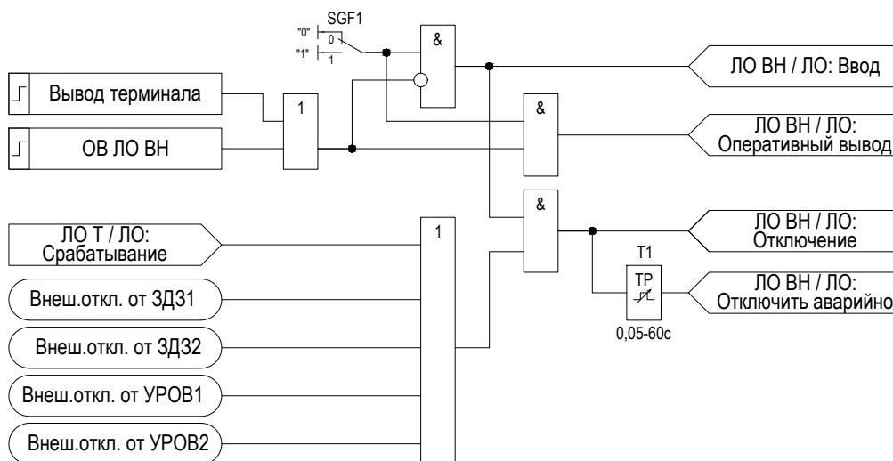
Рисунок 2.28 – Функциональная схема «ЛО»
