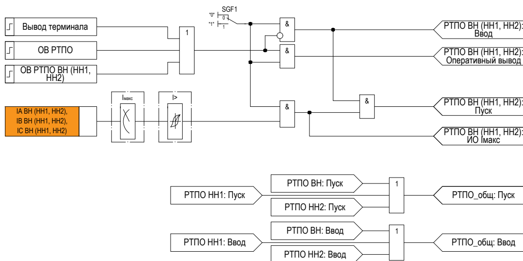
Рисунок 2.14 – Функциональная схема «РТПО»
